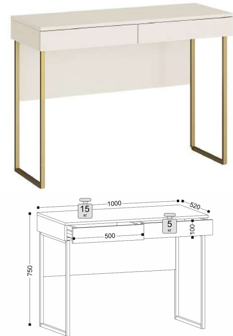
4 Стол ш-1000, г-520, в-750 труба 20x20
