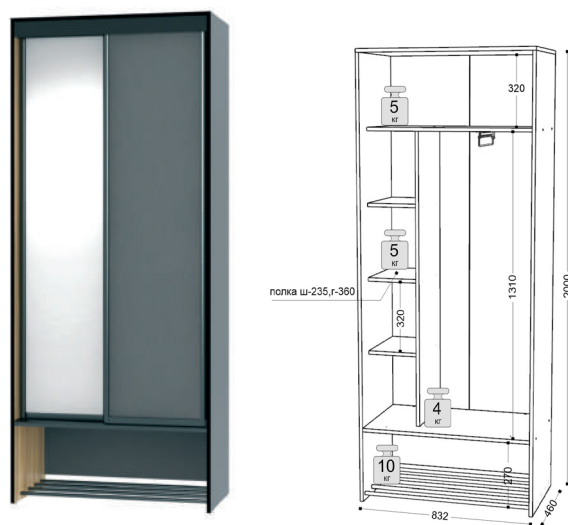
10 Шкаф-купе с зеркалом 10.1 Шкаф-купе без зеркала ш-832, г-460, в-2000
